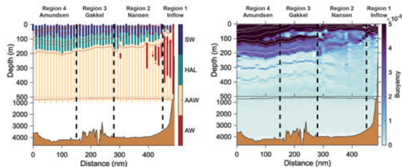
Figur 1: Tverrsnitt som viser vannmassetyper påvist langs det tverrfaglige transektet: SW = overflatevann, HAL = haloklin, AAW = arktisk atlantehavsvann, AW = atlantehavsvann.
