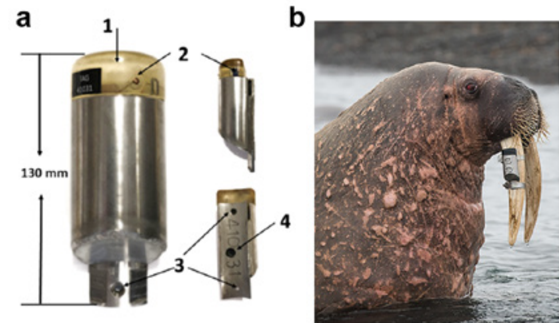
GPS-logger montert på hvalrossstann. Spesialdesignede GPS-sporingsenheter ble montert på støttennene til hvalrosser på Svalbard. a) GPS-loggeren sett forfra, fra siden og bakfra. 1: epoksyinnkapslet GPS; 2: saltvannsbryter; 3: skruehull; 4: kommunikasjonsport. b) Hvalross med en logger med ID D0. Bildet tatt ett år etter at enheten ble montert. Foto: Burney Iversen
