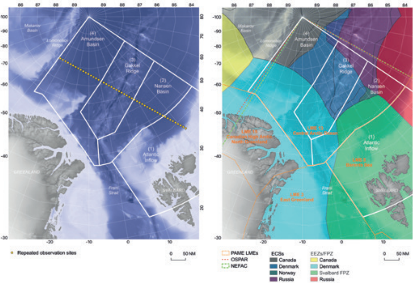
Kart 1: Batymetri- og observasjonssteder langs det tverrfaglige transektet. Figur: Paul A. Dodd / Norsk Polarinstitutt
