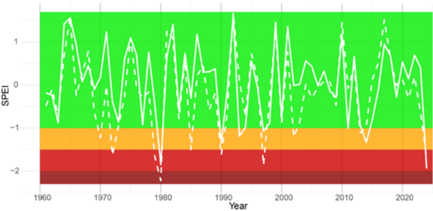
Evapotranspiration Index) for Øst-Finnmark for august (stiplet linje) og september (heltrukket linje). Tørkenivå indikeres med farge (oransje = moderat, rød = alvorlig, mørk rød = ekstrem). Merk at 1980 også var veldig tørt, men kaldere enn normalt, i motsetning til 2024. Graf: COAT
