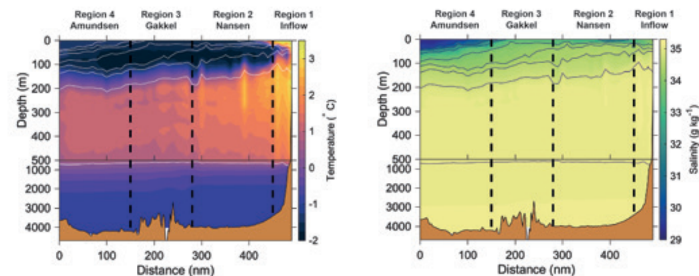
Figur 3: Tverrsnitt som viser temperatur (t.v.) og saltholdighet (t.h.) langs det tverrfaglige transektet.
